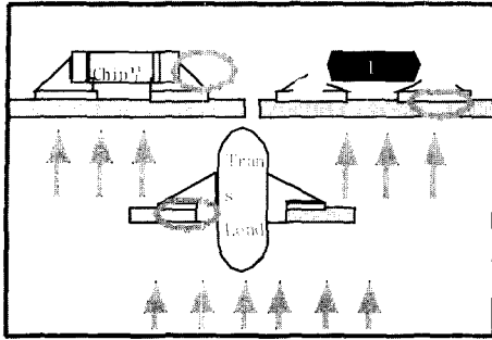
Fig. 9. Sn-0.5Cu-0.1Ni Soldering시 부품의 결정립 조대화 기구.
