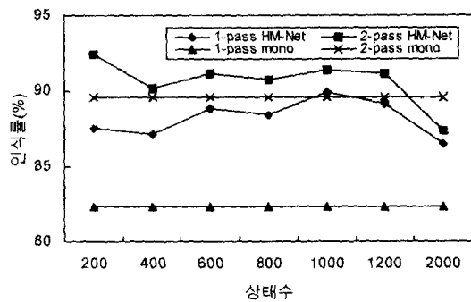
그림 7. 연속음성에 포함된 단어 인식률
