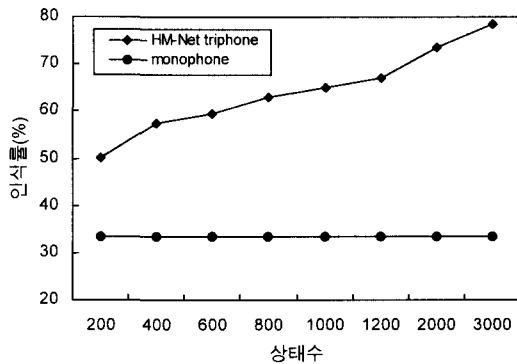
그림 4. 화자 독립 음소인식 실험결과
