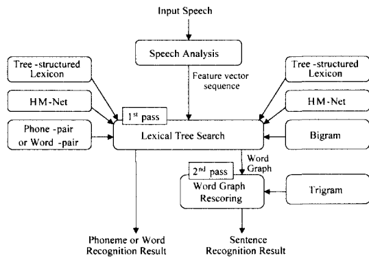
그림 3. 음성인식 시스템의 전체 구성도
