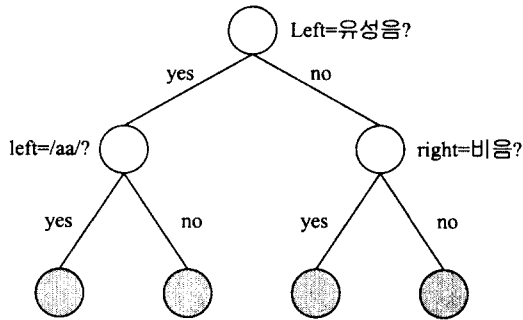
그림 2. 음소결정트리
