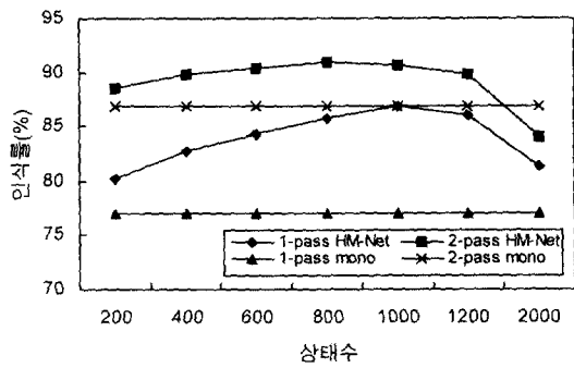
그림 6. 화자독립 연속음성인식률
