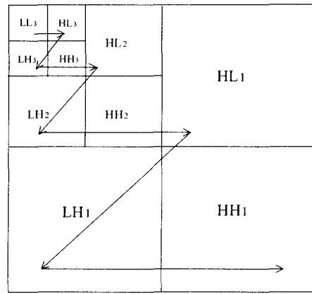
그림 5. 중요도에 따른 처리순서
