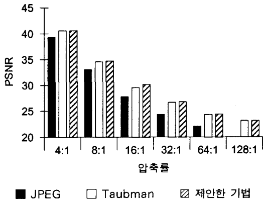
그림 21. 제안한 기법을 적용한 barbara 영상에 대한 PSNR 비교그래프
