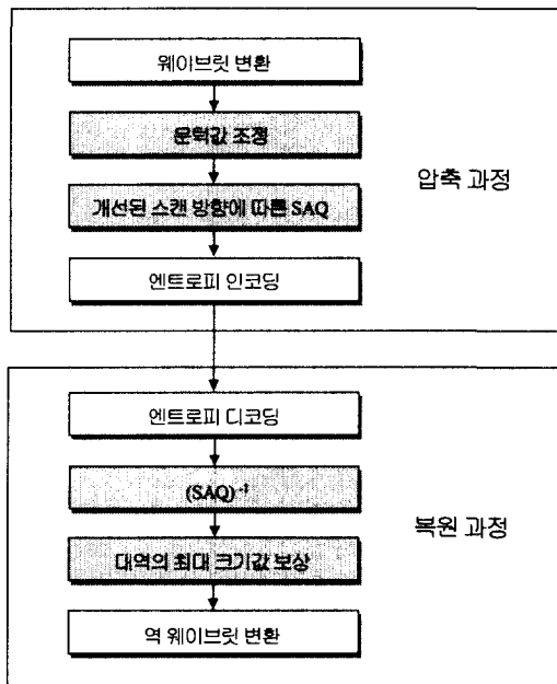
그림 8. 제안한 기법의 처리 단계
