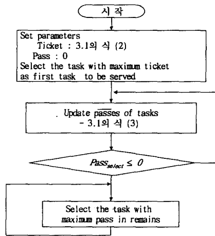
그림 1. MPSSA의 흐름도
