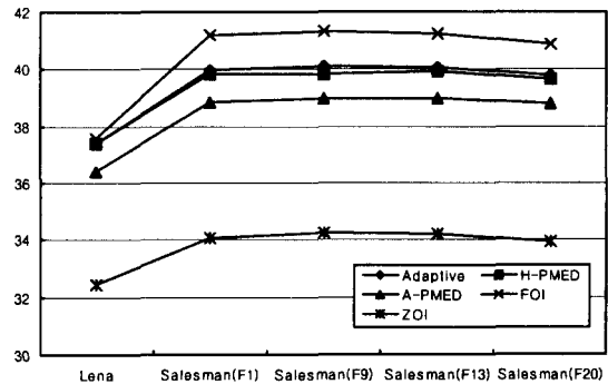
그림 5. Lena and Salesman의 PSNR
