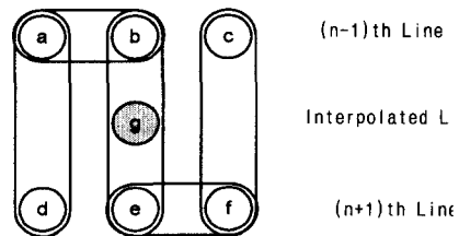
그림 2. 새로운 부윈도우 설정
