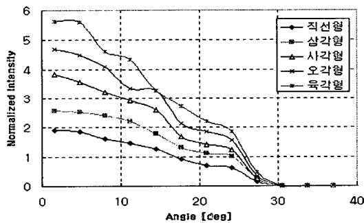
그림 4. 형태별 기본 배치에 따른 표준광도 Fig. 4. Normalized intensity according to basic arrangements by shape
