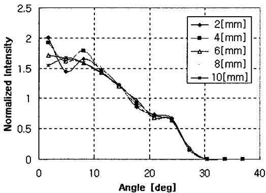
그림 9. 간격별 기본 배치에 따른 표준광도 Fig. 9. Normalized intensity according to basic arrangements by space
