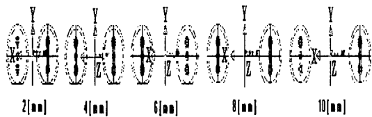
그림 8. 간격별 기본 배치 Fig. 8. Basic arrangements by LED lamps space
