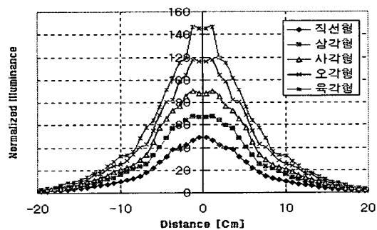
그림 5. 형태별 기본 배치에 따른 표준조도 Fig. 5. Normalized illuminance according to basic arrangement by shape
