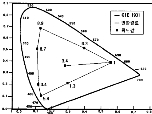
그림 14. 광색가변된 색좌표 및 휘도 Fig. 14. Chromaticity coordinates of the color & luminance of the LED lamps
