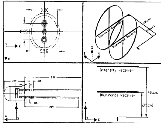
그림 1. 기준광원 Fig. 1. Standard source
