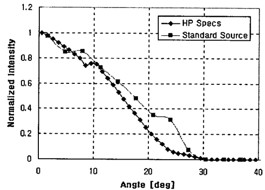
그림 2. HP Specs과 기준광원의 표준광도 Fig. 2. Normalized intensity of HP specs vs. standard source
