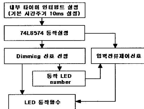
그림 13. 제어프로그램의 구성도 Fig. 13. Diagram of the control program
