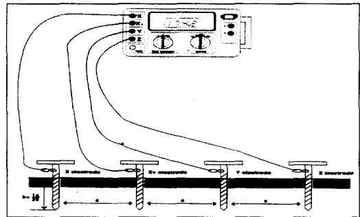
그림 1. 측정 탐침간의 구성도
