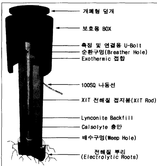
그림 4. XIT 접지시스템의 기본 구조
