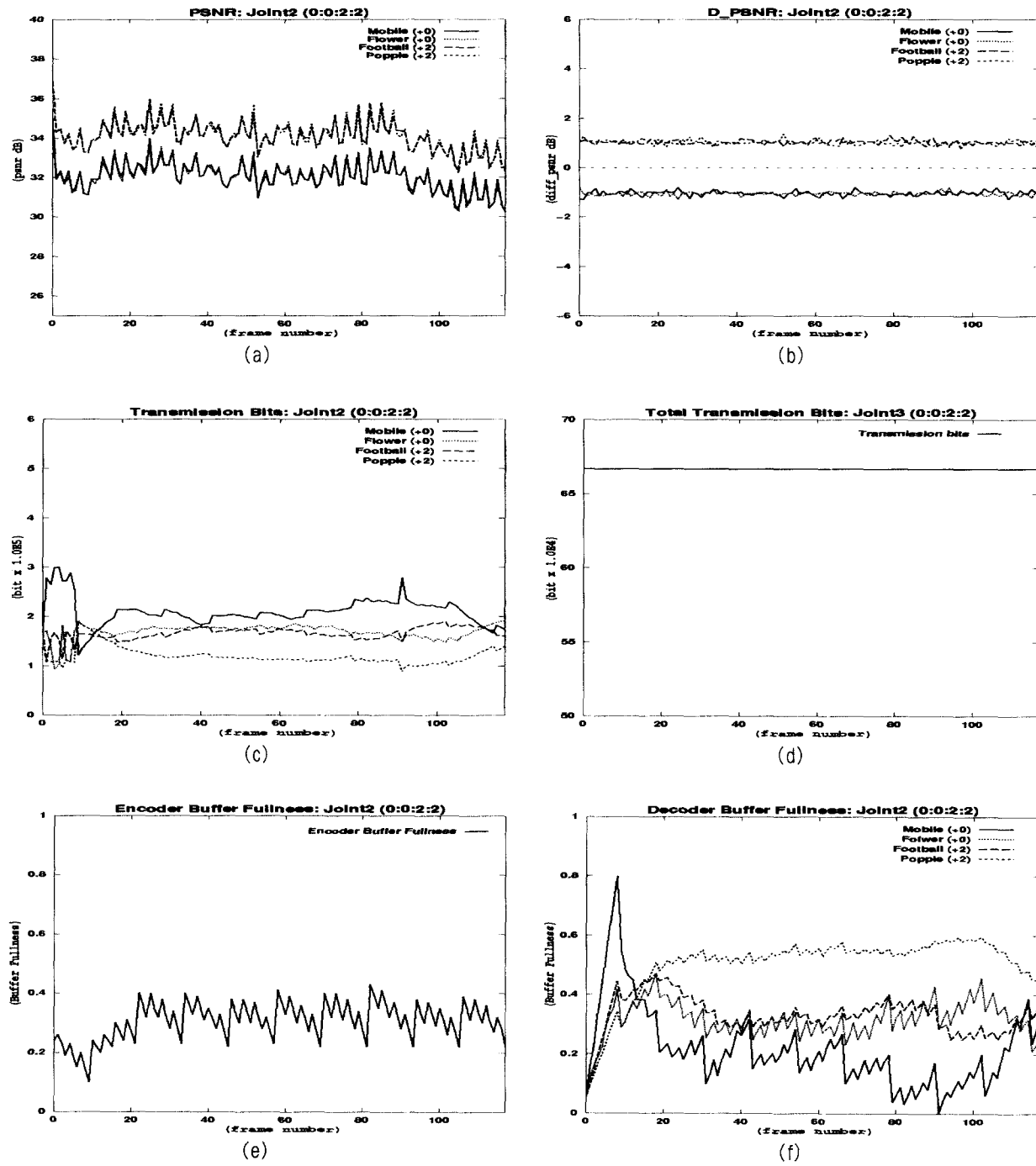
그림 8. 선택적 화질 제어 결과 ( \Delta PSNR=0:0:2:2): (a) PSNR, (b) diff_PSNRk, (c) 개별 전송 비트량, (d) 전체 전송 비트량, (e) 공통 부호기 버퍼 상태, (f) 개별 복호기 버퍼 상태
