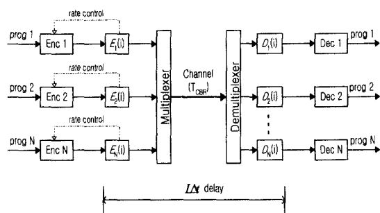
그림 1. 독립 부호화 시스템 Fig. 1. Independent coding system
