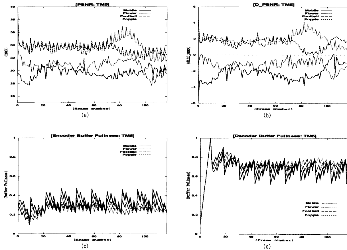
그림 6. 독립부호화 결과 (a) PSNR, (b) diff_PSNR, (c) 부호기 버퍼 상태, (d) 복호기 버퍼 상태 Fig. 6. independent coding results: (a) PSNR, (b) diff_PSNR, (c) encoder buffer status, (d) decoder buffer status
