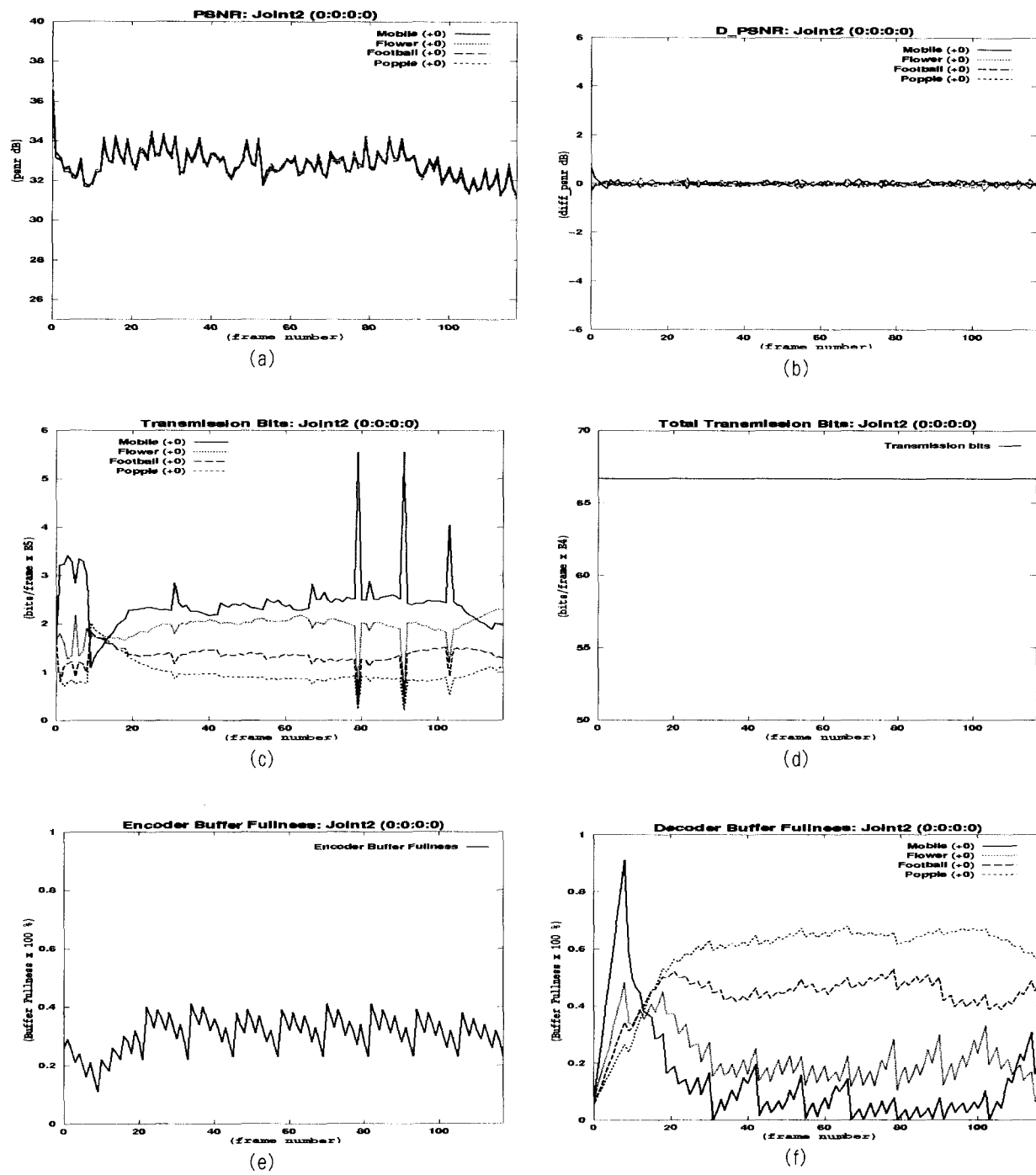
그림 7. 선택적 화질 제어 결과 ( \Delta\text{PSNR}=0:0:0:0 ): (a) PSNR, (b) diff_PSNRk, (c) 개별 전송 비트량, (d) 전체 전송 비트량, (e) 공동 부호기 버퍼 상태, (f) 개별 복호기 버퍼 상태
