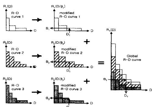
그림 5. 선택적 화질 제어를 위한 비트량 할당 방식 Fig. 5. Bit allocation method for selective quality control
