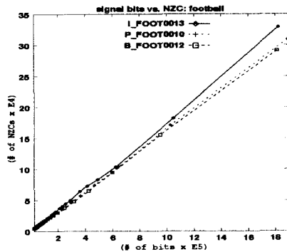
그림 3. QP를 1에서 31로 변화시킬 때 I, P, B 픽처의 프레임 당 발생하는 비트 수와 NZC 수의 관계 Fig. 3. Relationship between the number of NZCs and the number of bits generated per frame as the QP is increased from 1 to 31 for I-, P-, B-picture
