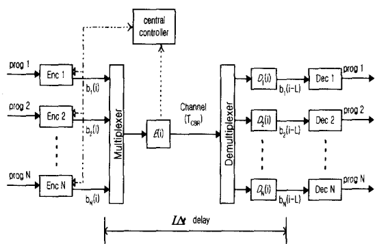
그림 2. 선택적 화질제어 시스템 Fig. 2. Selective quality control system
