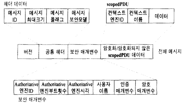
(그림 3) SNMPv3 메시지 구조
