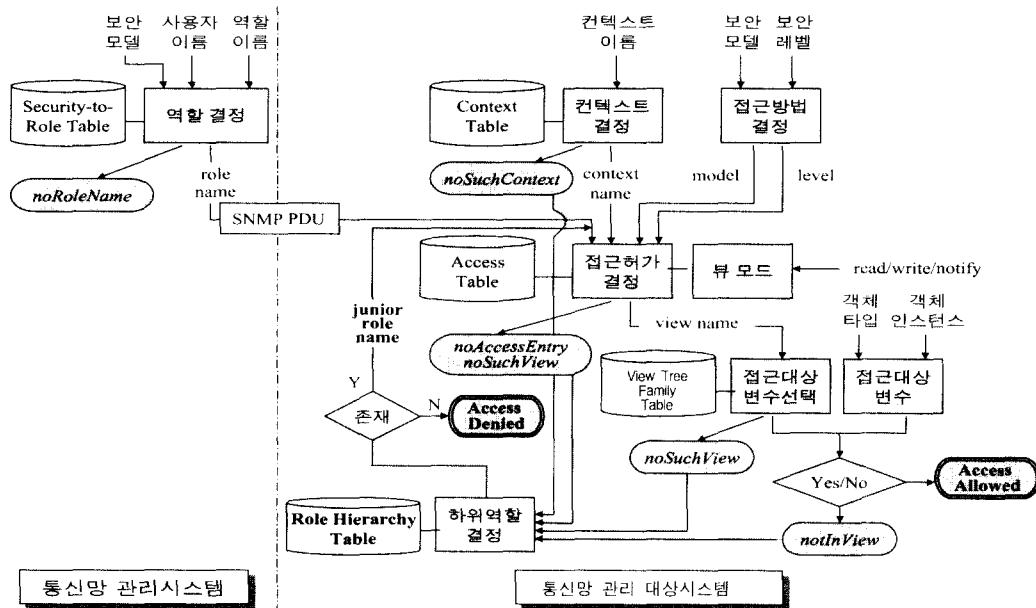
(그림 8) 역할기반 보안관리 모델을 적용한 뷰기반 접근통제 절차
