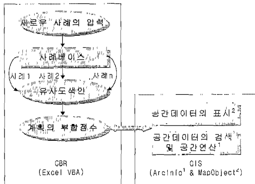
[그림 3] 추론 시스템의 구조
