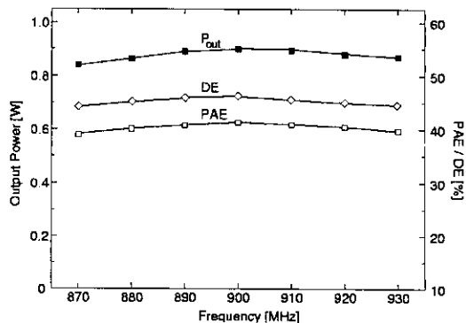
그림 11. 공급 전압이 1.8V일 때 주파수에 따른 출력 전력, 드레인 효율, PAE
