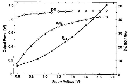
그림 10. 공급 전압에 따른 출력 전력, 드레인 효율, PAE
