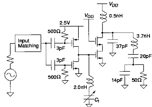
그림 8. Class-E 전력 증폭기의 회로도
