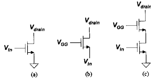
그림 7. (a) 통상의 common-source 스위치 (b) common-gate 스위치 (c) cascode 스위치
