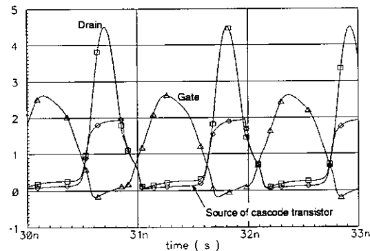
그림 6. 전력 증폭기의 모의 실험 파형
