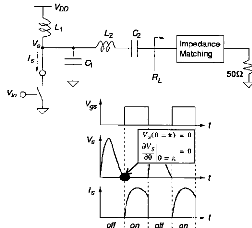
그림 4. Class-E 전력 증폭기와 전압 및 전류 파형
