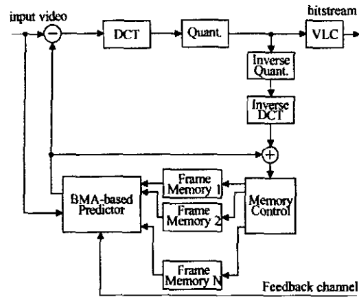
그림 1. 다중 레퍼런스 프레임 기반의 동영상 부호화 구조
