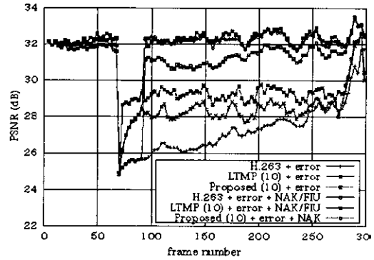
그림 7. "Foreman" 영상에서 두 개의 GOB 손실시 NAK와 결합했을 때 PSNR 성능
