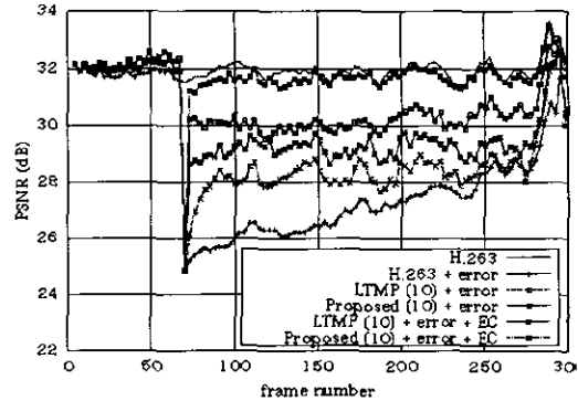
그림 4. "Foreman" 영상에서 두 개의 GOB 손실시 EC와 결합했을 때 PSNR 성능
