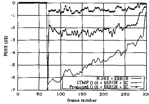
그림 5. "Foreman" 영상에서 두 개의 GOB 손실시 EC와 결합했을 때 원영상과의 PSNR 차
