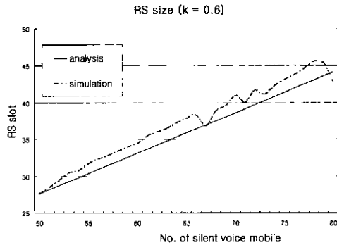
그림 6. 예약슬롯 크기
