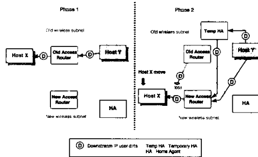
그림 5. 경로 최적화를 사용한 Mobile-IPv6 핸드오프 동안 사용자 데이터 전송
