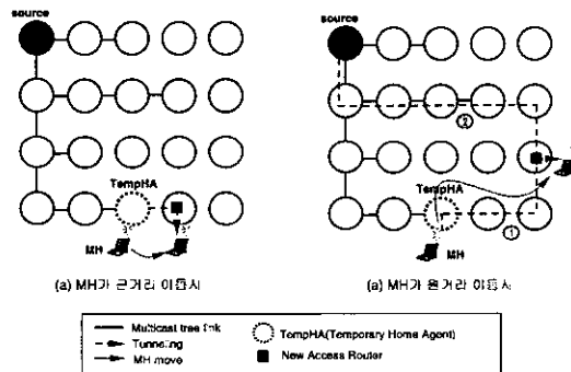
그림 6. 핸드오프 기반 멀티캐스트 기법
