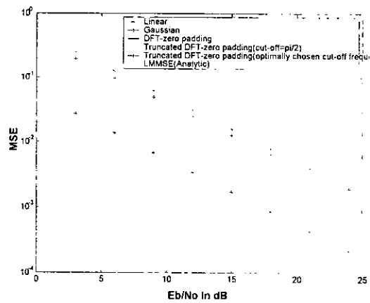
그림 10. P=6 일 때 주파수 영역 채널 추정에서 여러 내삽 방법에 대한 평균 제곱 오차 비교
