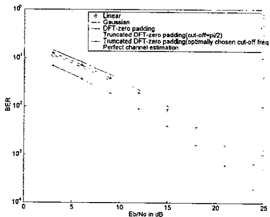
그림 11. P=6 일 때 주파수 영역 채널 추정에서 여러 내삽 방법에 대한 비트 오류율 비교
