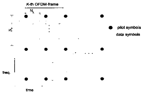
그림 3. k번째 OFDM 프레임에서 파일럿 심볼 배열
