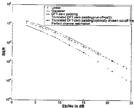
그림 9. P=12 일 때 주파수 영역 채널 추정에서 여러 내삽 방법에 대한 비트 오류율 비교
