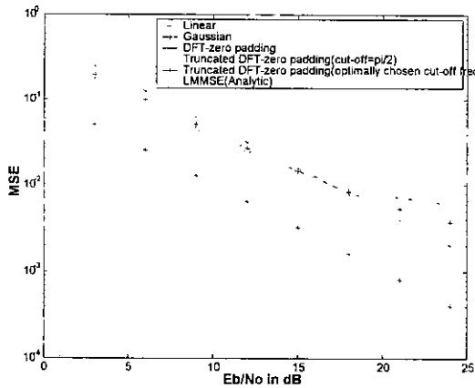
그림 8. P=12 일 때 주파수 영역 채널 추정에서 여러 내삽 방법에 대한 평균 제곱 오차 비교
