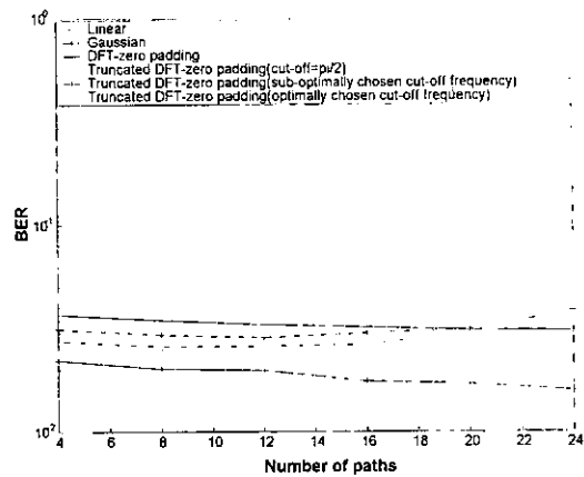
그림 13. E_b/N_0=10dB 일 때 경로 수에 따른 여러 채널 추정 방법들의 비트 오류율
