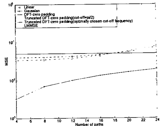
그림 7. E_b/N_0=10\text{dB} 일 때 다중 경로 수에 따른 여러 채널 추정 방법의 평균 제곱 오차 계산
