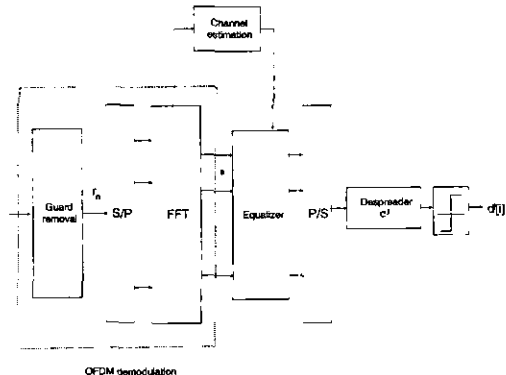
그림 2. OFDM-CDMA 수신기 블록 모형도
