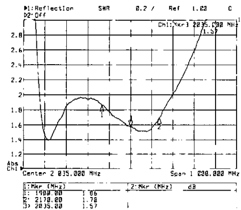
그림 4.3 제작된 안테나의 VSWR
