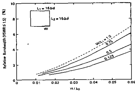
그림 2.3 단락판 폭이 L₁보다 작을 때의 대역폭 변화
