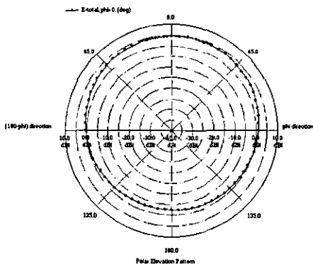
(b) 수평패턴
