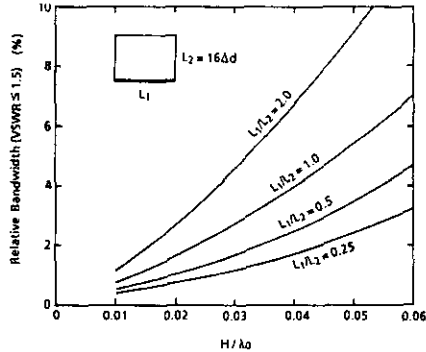
그림 2.2 단락판 폭이 L₁과 같을 때의 대역폭 변화
