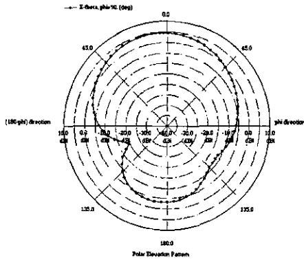
(a) 수직패턴
