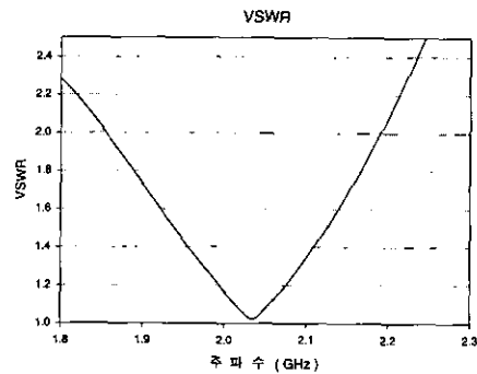
(b) VSWR
