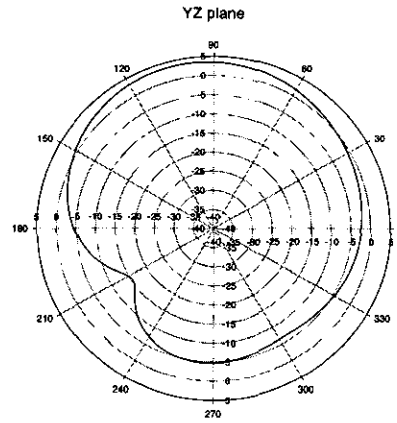
(a) 수직 패턴
