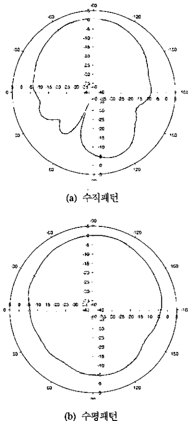
그림 4.2 제작된 PIFA의 복사 패턴 (단위 : dBd)
