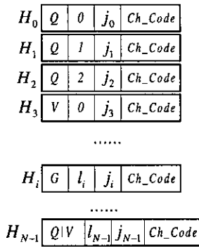
그림 8. 순방향 추적 이력 정보 데이터의 구조
