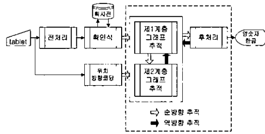
그림 9. 제안된 알고리즘을 이용한 온라인 문자인식 시스템의 구성
