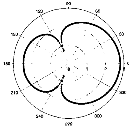
그림 4a. Bow-tie 안테나의 자유공간 방사특성; \phi = 0^\circ
