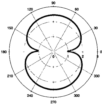
그림 4b. Bow-tie 안테나의 자유공간 방사특성; \theta=90^\circ
