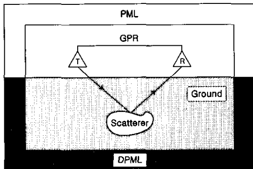
그림 2. 지면 위에서의 레이더 탐색 구성
