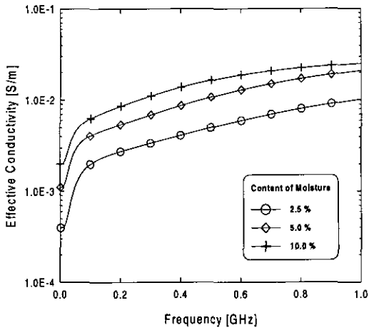
그림 1b. 수분 함유량 및 주파수 변화에 따른 지하매질의 실효 도전율 변화도
