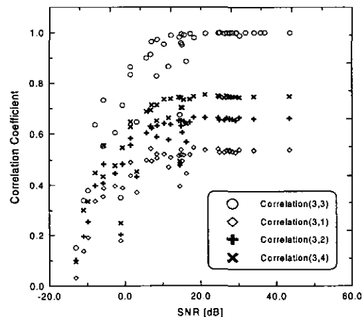
그림 8. 동일한 지하에 매설된 산란체 사이의 상관계수
