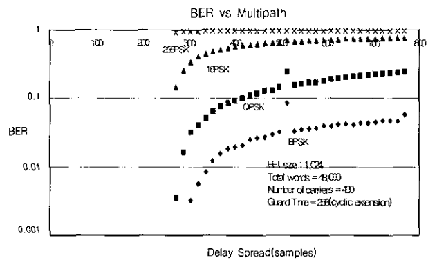
(그림 6) 지연확산 대비 비트에러율
