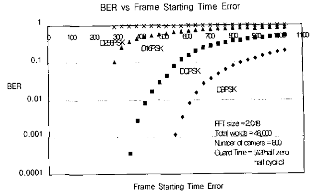
(그림 9) 프레임 타이밍 오차 대비 비트에러율
