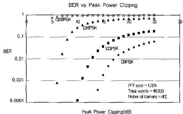
(그림 7) 최대전력 클리핑 대비 비트에러율
