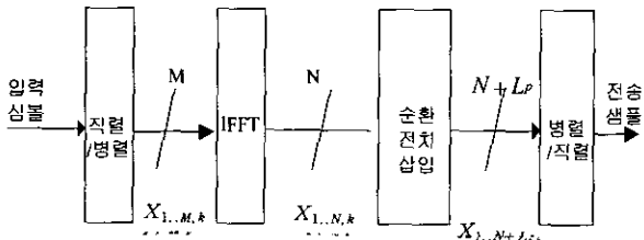
(그림 2) OFDM 송신부의 블록도
