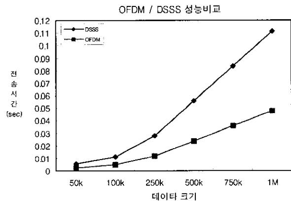
(그림 11) OFDM/DSSS 성능 비교
