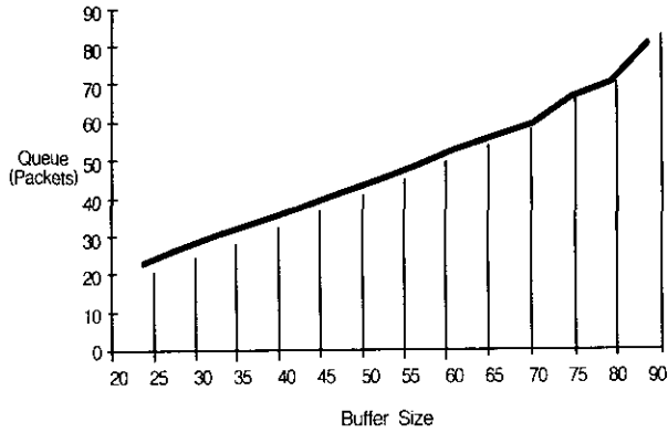
(그림 3) DT의 버퍼 크기에 따른 큐 특성
