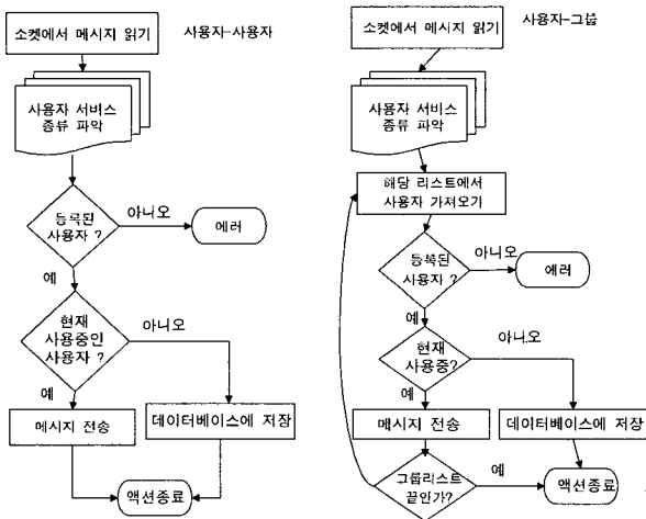
(그림 12) 메시지 전송 알고리즘
