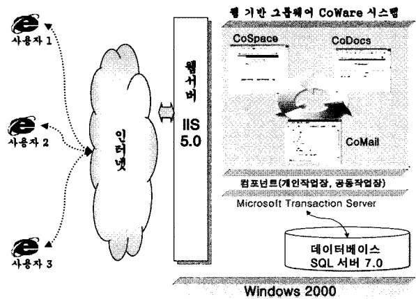
(그림 1) CoWare 시스템 동작환경
