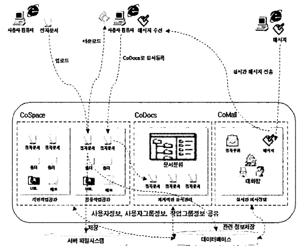
(그림 16) CoWare 사용 시나리오
