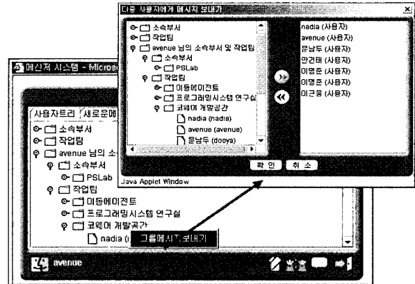
(그림 14) 다중 선택 메시지 전송
