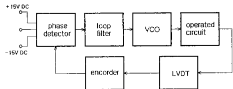
그림 5. PLL의 블록도. Fig. 5. Block diagram of PLL.
