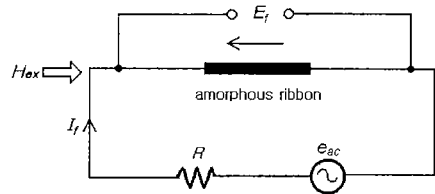
그림 8. MI 효과의 측정회로. Fig. 8. Circuit for measuring MI effect.
