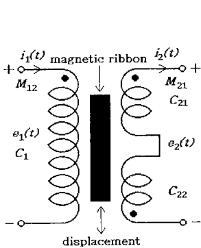
그림 3. LVDT의 설명도. Fig. 3. Schematic illustration of LVDT.
