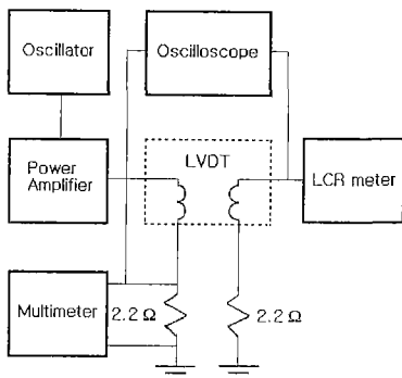
그림 11. 변위센서의 측정시스템.
