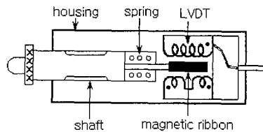
그림 2. 변위센서의 구성도.
