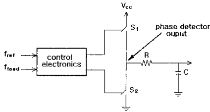
그림 6. 위상주파수 검파기의 등가회로. Fig. 6. Equivalent circuit of phase frequency detector.
