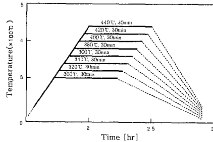
그림 1. 열처리온도 스케줄.
