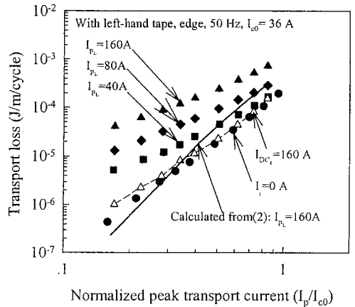
그림 5. 좌측 테이프의 각종 교류 전류에 대한 통전 손실 - 정규화된 피크 통전전류(가장자리 전압리드를 사용).
