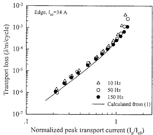
그림 3. 통전전류의 각종 주파수에 대한 통전손실 - 정규화된 피크 전류(가장자리 전압리드 사용).
