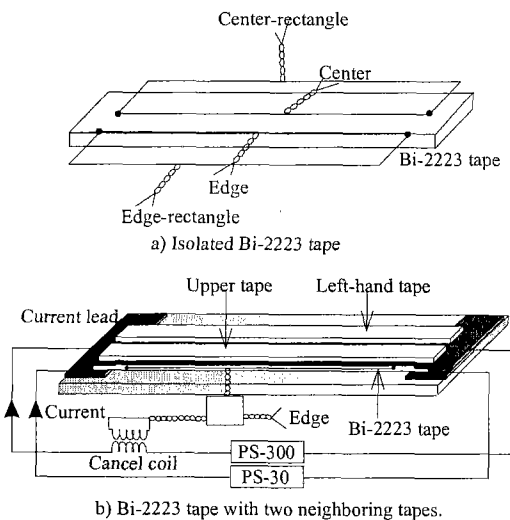
그림 1. 시료의 개략도.
