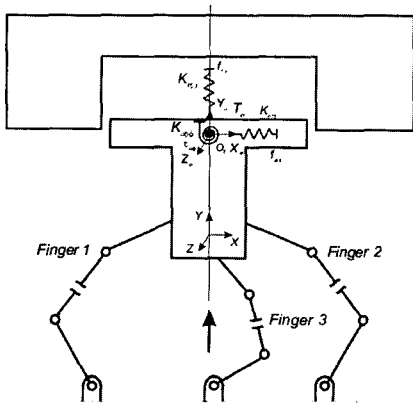
그림 2. 로봇 손을 이용한 T형 물체의 조립 작업. Fig. 2. Assembly task of T-type object by robot hands.
