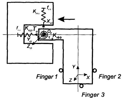
그림 4. 로봇 손을 이용한 7형 물체의 조립 작업. Fig. 4. Assembly task of 7-type object by robot hands.
