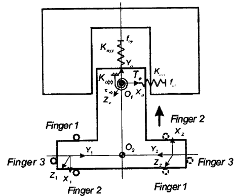
그림 6. 로봇 손을 이용한 \perp 형 물체의 조립 작업. Fig. 6. Assembly task of \perp -type object by robot hands.
