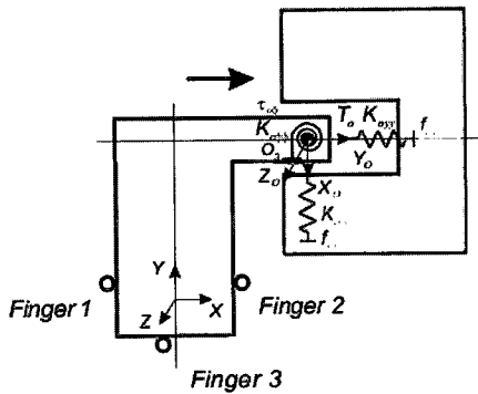
그림 5. 로봇 손을 이용한 \Gamma 형 물체의 조립 작업. Fig. 5. Assembly task of \Gamma -type object by robot hands.
