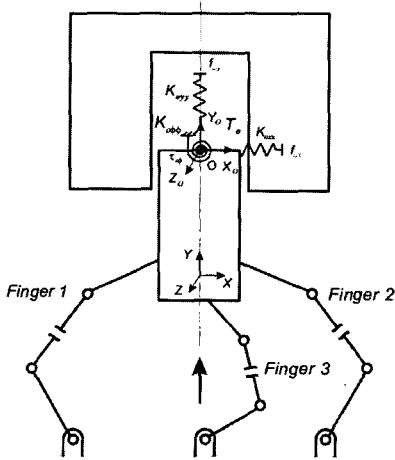
그림 1. 로봇 손을 이용한 물체의 조립 작업. Fig. 1. Assembly task of an object by robot hands.
