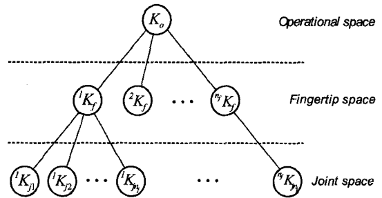
그림 3. 로봇 손을 이용한 물체의 조작을 위한 강성 관계.
