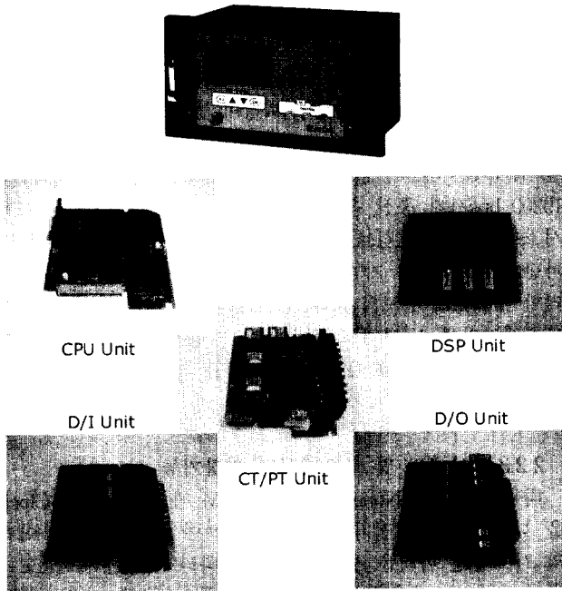
그림 3. 개발된 디지털 보호계전기의 외형 및 내부 모듈
