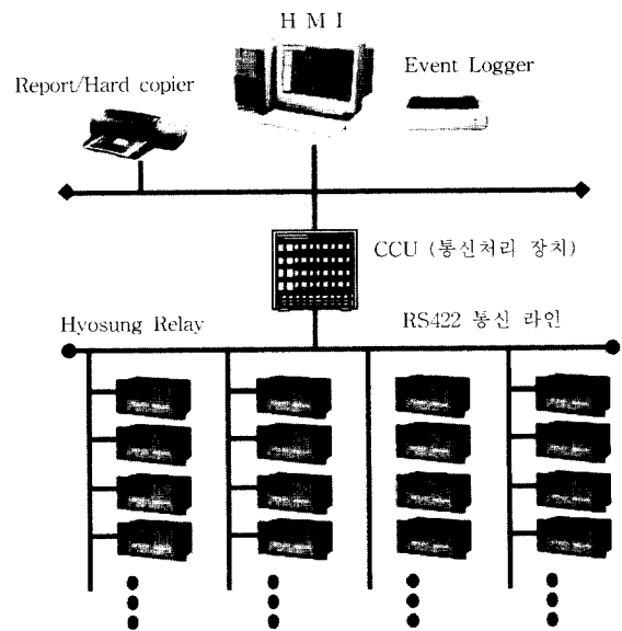
그림 5. 시스템 구성도
