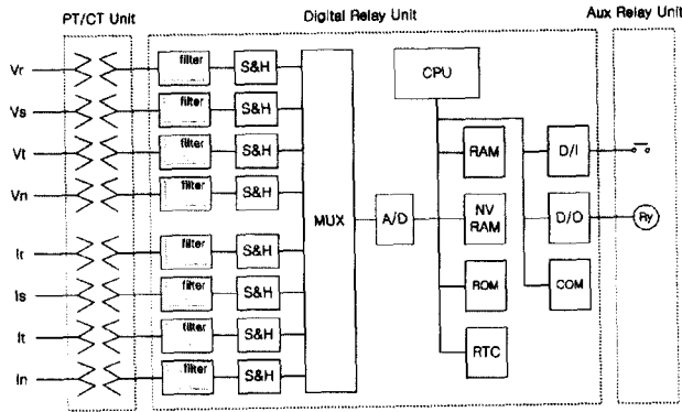
그림 1. 디지털 보호계전기의 구성
