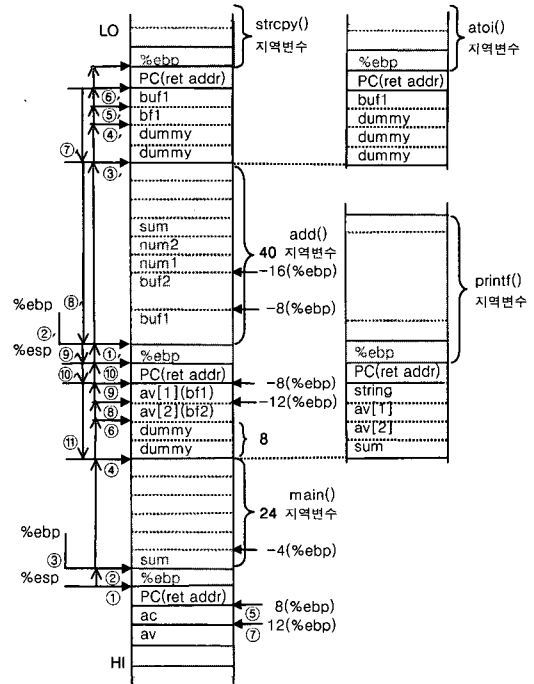
(그림 5) (프로그램 3)의 진행에 따른 스택 변화과정
