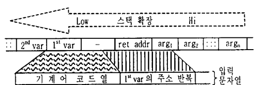
(그림 9) 버퍼넘침을 유도하는 입력문자열의 구성
