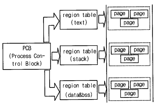
(그림 1) 실행파일 이미지의 구성
