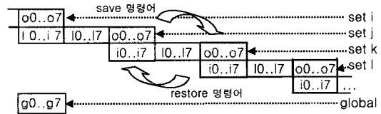
(그림 7) 스파크 프로세서의 다중 레지스터 개념
