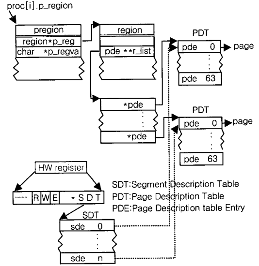
(그림 2) 실행파일을 위한 메모리 관리구조
