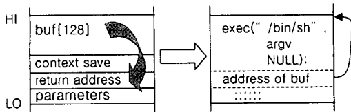
(그림 4) 의도적인 버퍼넘침의 유도
