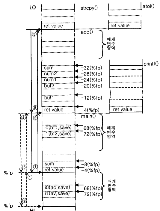
(그림 8) (프로그램 5)의 진행에 따른 스택 변화과정
