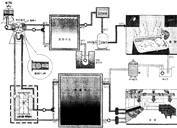
〈그림 32〉생활배수열의 히트펌프 시스템 기본구성도
