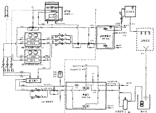
[그림 5.1] 온천숙박시설에 대한 수축열식 히트펌프 시스템 구성도
