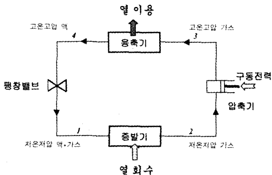
<그림 3.1>히트 펌프 기본 원리도
