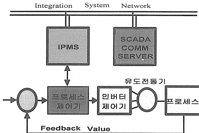
(그림 2.9) SCADA와 IIMS의 I/F 구성도
