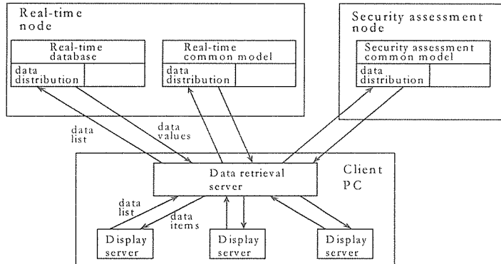
(그림 2.5) Data Retrieval Server 구성도
