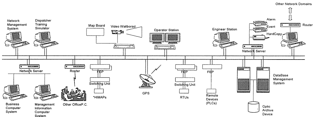
(그림 2.2) 전체시스템 구성도
