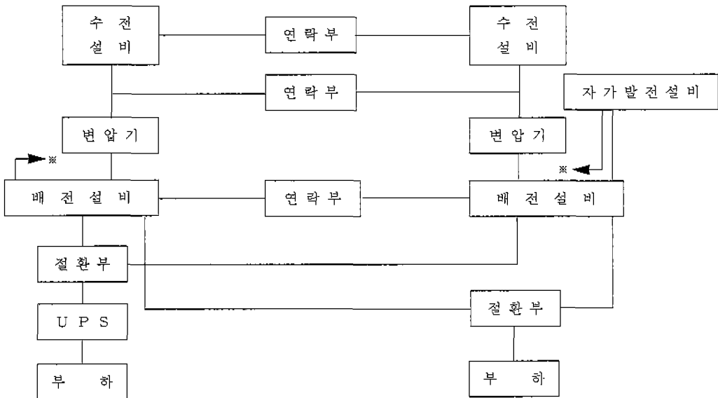
그림 1 전원시스템의 신뢰도 향상을 위한 단선도
