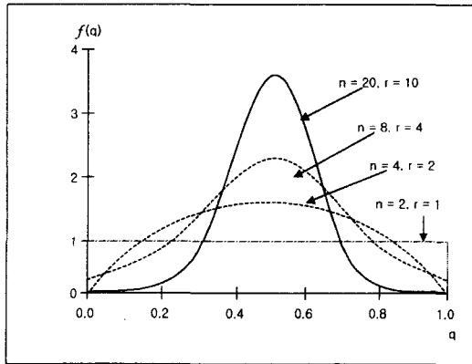
〈그림-1〉 대칭적 beta 분포
