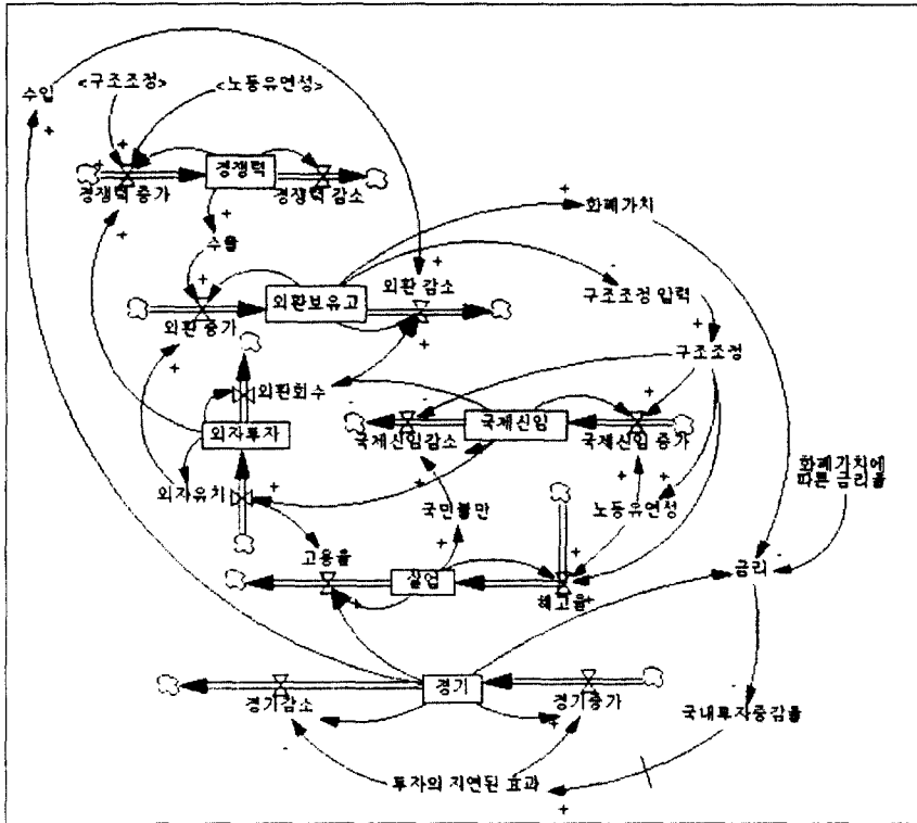
<그림 5> 김대중 대통령 인지도의 시뮬레이션 모델
