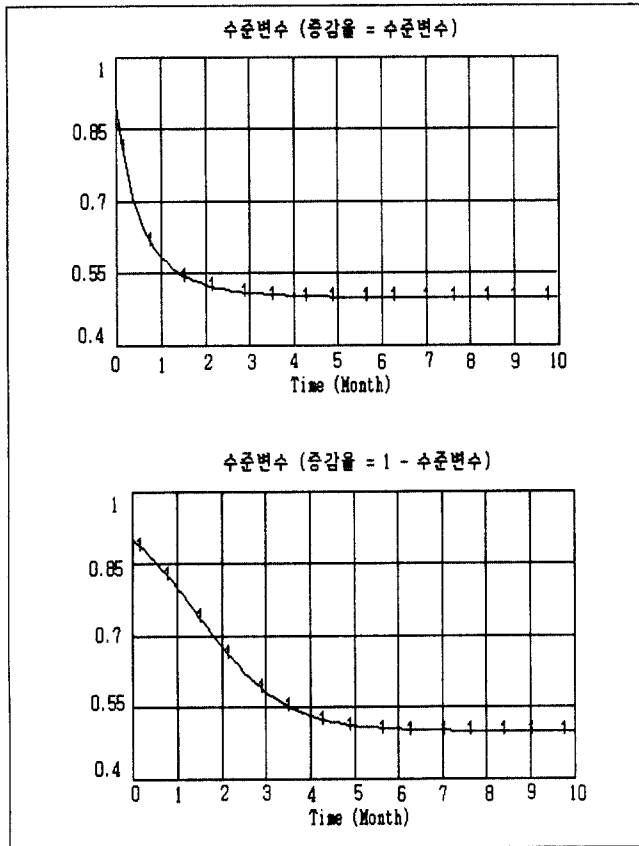
<그림 3> 수준변수의 초기값을 높게 설정하였을때의 형태
