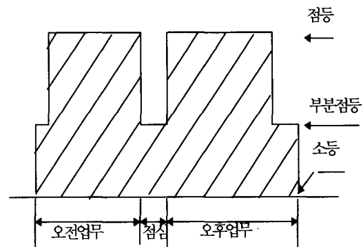
그림 4. 건물 사용 스케줄에 의한 조명제어
