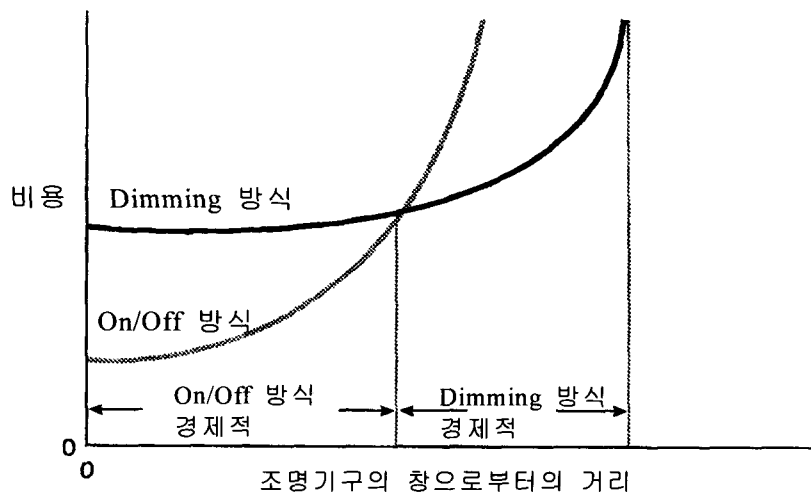
그림 6. 점멸제어(On/Off)와 조광제어(Dimming)의 경제성비교
