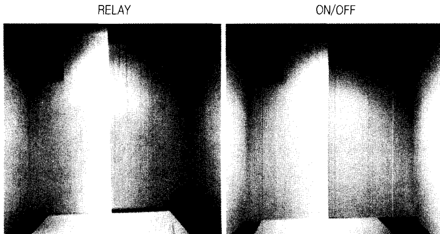
그림 11. Radiance 컴퓨터 시뮬레이션에 의한 결과의 정확성 검증
