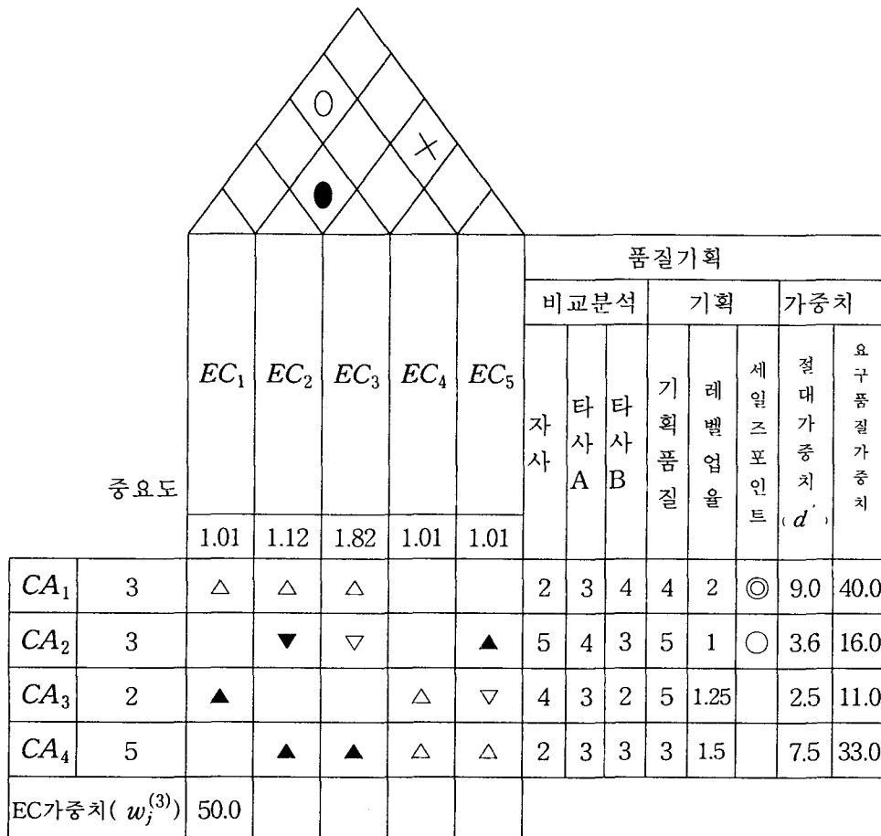
[그림 3.3] 식(3.4)을 이용한 EC 가중치 계산
