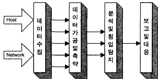
그림 2. 침입 탐지 시스템의 기술적 구성요소 Fig. 2. Technical constituent of IDS.
