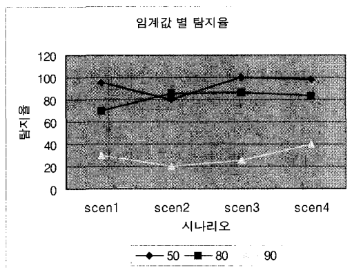
그림 11. 임계값 별 침입 탐지율 변화 Fig. 11. Intrusion detection ratio variation following by critical value.
