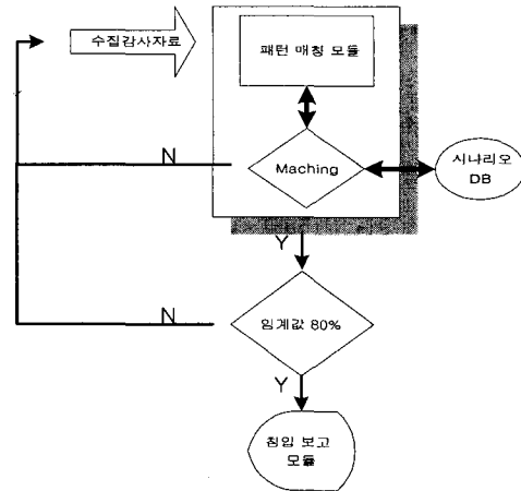
그림 10. 침입 판단 구조도 Fig. 10. Intrusion decision structure.
