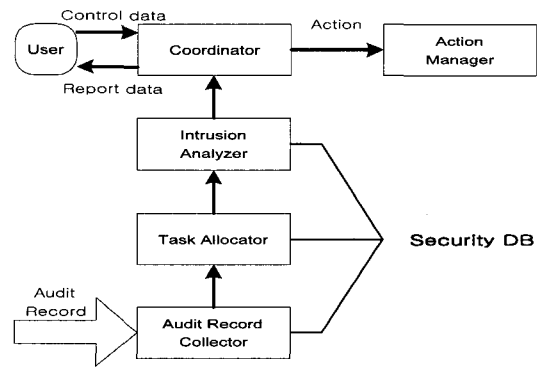
그림 3. 실시간 침입 탐지 시스템 구조 Fig. 3. Frame of real time IDS.
