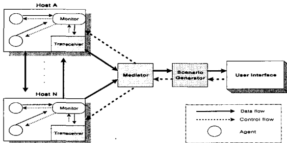
그림 5. 제안된 패턴 추출 에이전트 침입 탐지 시스템 모델 Fig. 5. Suggested pattern extracting agent IDS model.
