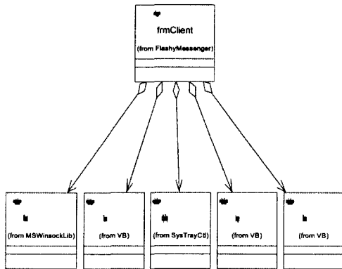
그림 5. Client Class 다이어그램
