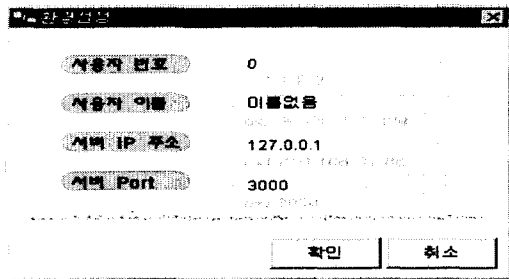
그림 12. 환경설정 화면
