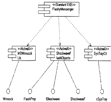
그림 7. Component 다이어그램
