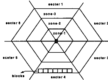
그림 1. 시스템 모델
