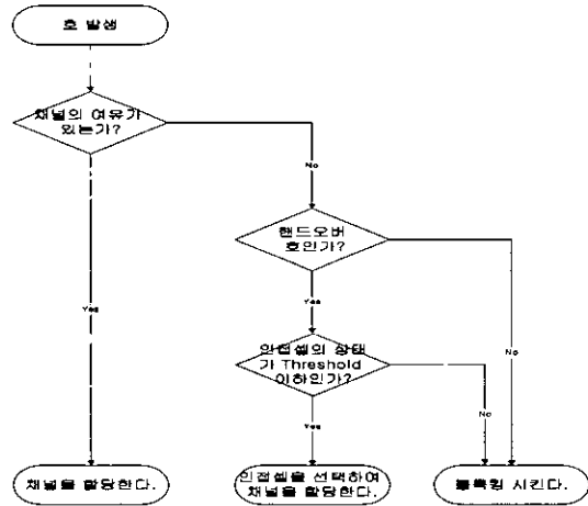
그림 6. 채널차용 알고리즘
