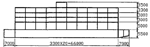
Fig. 7 Longitudinal section
