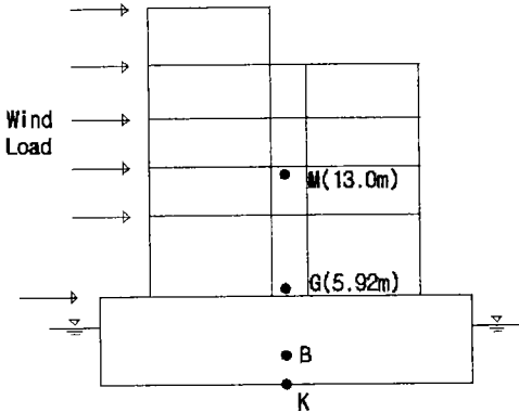
Fig. 6 Metacenter
