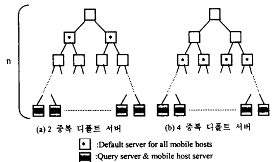
그림 5. 이진 트리에서의 중복 디폴트 서버 구조
