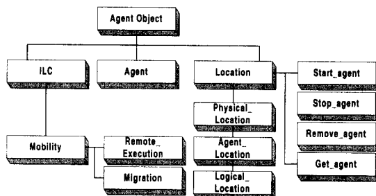
그림 3. 이동에이전트의 자바클래스 상속구조
