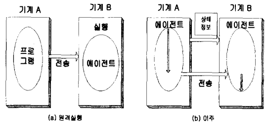
그림 1. 이동성의 두 가지 방법
