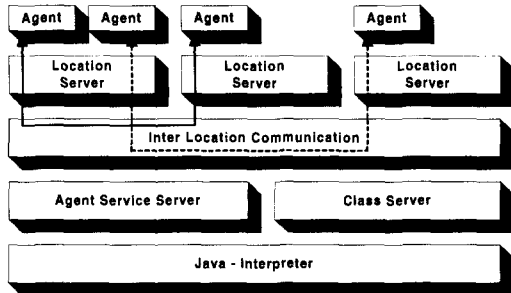
그림 5. 이동에이전트 시스템 하부구조
