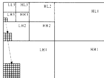
그림 3. 각 부밴드별 벡터 크기
