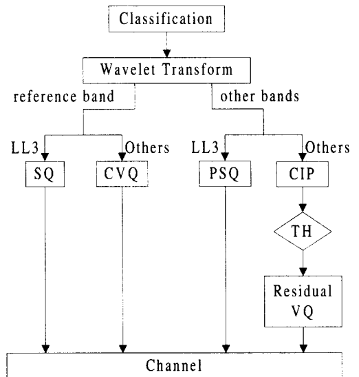
그림 1. 제안된 방법의 블록선도
