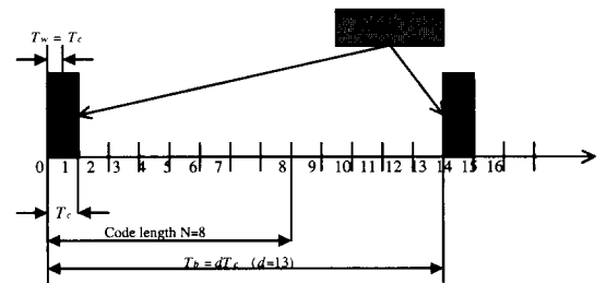
그림 1. 다파장 OCDMA 네트워크 송신자의 신호 주기 (N=8, d=13의 경우)
