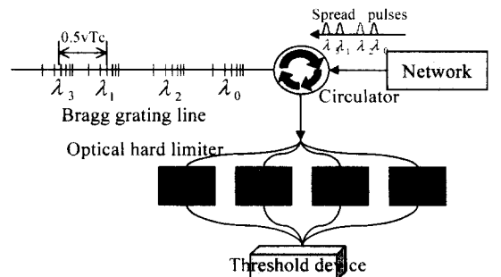
그림 3. 광 영역에서 구현된 OCDMA 복호기
