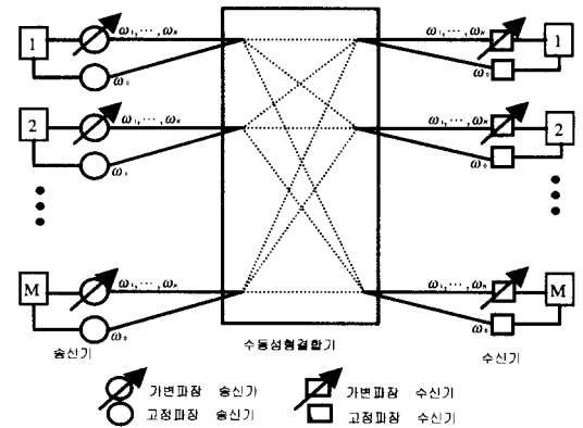
그림 1. 수동성형 결합기를 사용한 망의 구조
