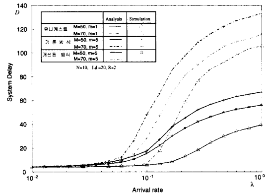
그림 6. 사용자 수 변화에 따른 도착율 대 시스템 지연특성
