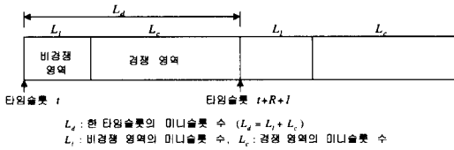
그림 3. 제어채널 구성
