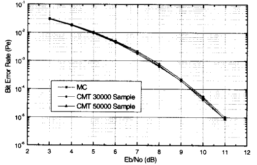
(b) TWTA의 input back-off가 -1dB 일 때
