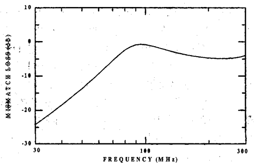
그림 3. AB단자에서 발룬과 안테나 입력간에 부정합 손실 ( Z_{AB} = 100 \Omega )
