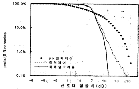
그림 7. 전력제어에 따른 신호대 잡음비 오류 분포
