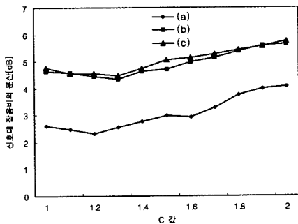
그림 10. C값에 따른 신호대 잡음비의 분산 변화 (a) 10km/h (b) 50km/h (c) 100km/h
