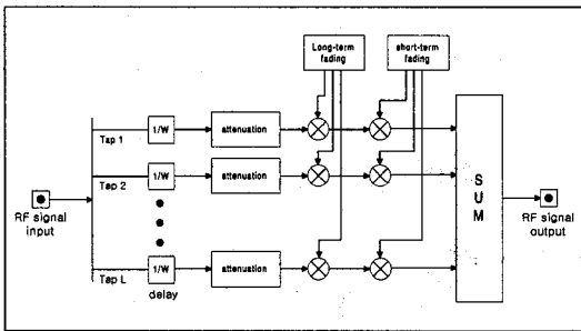
그림 2. 채널 블록도
