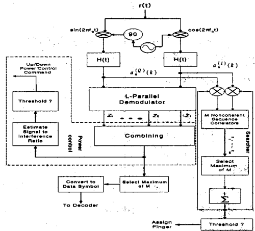
그림 3. 모의실험 역방향 수신기
