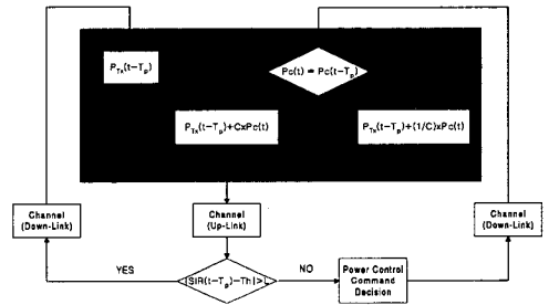
그림 4. 적응 알고리즘 전력제어 흐름도
