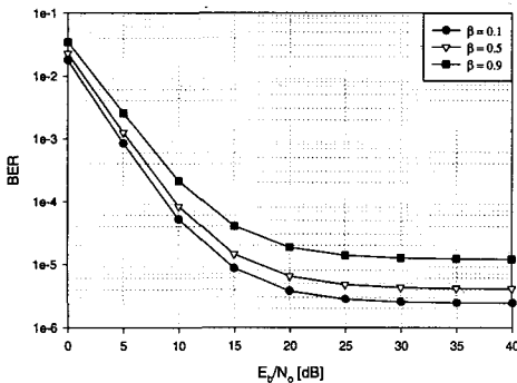
그림 5. 주파수 선택성 다중경로 페이딩 채널 특성(β)에 따른 Multi-Carrier CDMA 시스템의 오율 성능 (다중사용자 수=26, Multi-Carrier의 수=127, 다중사용자 간섭분포 : Case I, RAKE 수신기의 가지수=4 )
