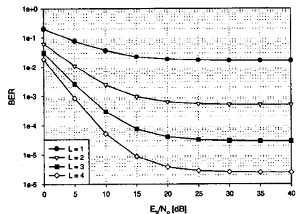
그림 4. 주파수 선택성 다중경로 페이딩 채널에서 RAKE 수신기의 가지수에 따른 Multi-Carrier CDMA 시스템의 오율 성능 ( \beta = 0.3 , 다중사용자 수=26, Multi-Carrier의 수=127, 다중사용자 간섭분포 : Case I)
