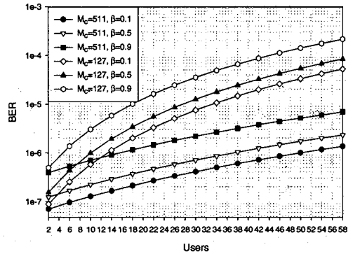
그림 9. 주파수 선택성 다중경로 페이딩 채널 특성과 다중사용자 수에 따른 Multi-Carrier CDMA 시스템의 오율 성능 ( E_b/N_0=15 [dB], 간섭분포: Case III, RAKE 수신기의 가지수=4, Multi-Carrier의 수=127)
