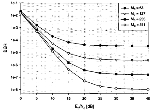
그림 6. 주파수 선택성 다중경로 페이딩 채널에서 Multi-Carrier의 수에 따른 Multi-Carrier CDMA 시스템의 오율 성능 (β = 0.1, 다중접속 사용자수=26, 다중사용자 간섭분포 : Case I, RAKE 수신기의 가지수 = 4 )
