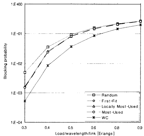
그림 6. 양방향 5 × 5 매쉬-토러스 망에서의 P_b vs. 부하
