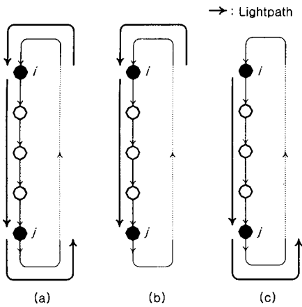
그림 2. 단방향 링 망에서 파장 \lambda_m 의 부분적인 사용 집중화 (packing) 현상
