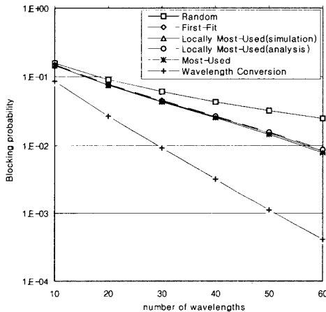
그림 4. 양방향 5 × 5 매쉬-토러스 망에서의 P_b vs. 파장의 개수; 부하/파장링크 = 0.625 [Erlangs]
