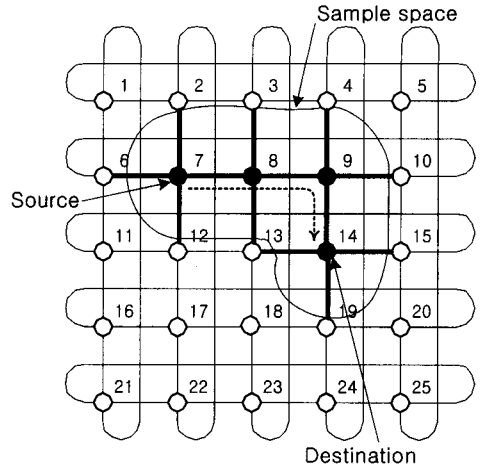
그림 1. 5 × 5 양방향 매쉬-토러스 망에서 라우팅 경로 주변의 샘플 공간의 예
