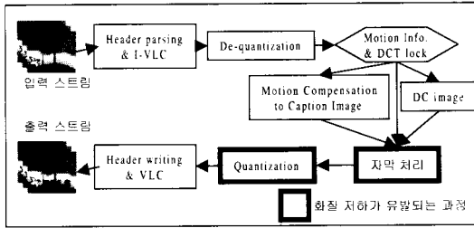
그림 4 MC-DCT 영역에서의 자막 처리 과정
