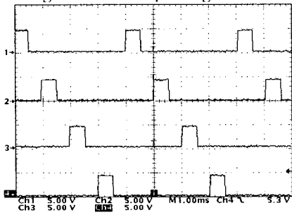
(d) Each gate signals
