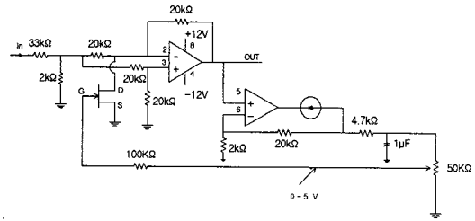
그림 6. AGC 회로도 Fig. 6. AGC circuit.
