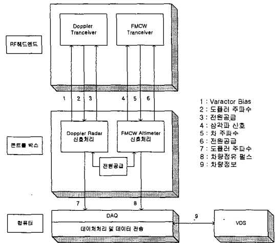
그림 2. 레이더방식 차량감지기 시스템의 전체 구성도 Fig. 2. Full topology of radar vehicle detector system.
