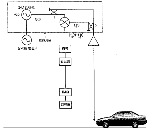
그림 4. FMCW 고도계의 블록도 Fig. 4. The block diagram of FMCW altimeter system.
