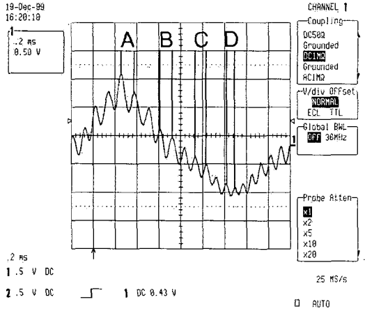
그림 12. 차 신호의 일차 증폭후의 신호를 디지털 오실로스코프로 찍은 파형
