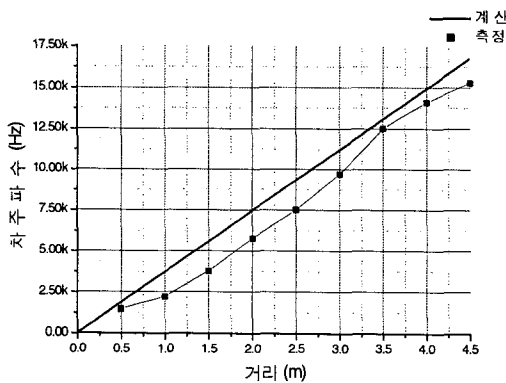
그림 11. 거리에 따라 측정된 차 주파수
