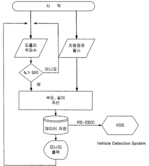
그림 9. 데이터처리 프로그램 흐름도 Fig. 9. Flow chart for data management.
