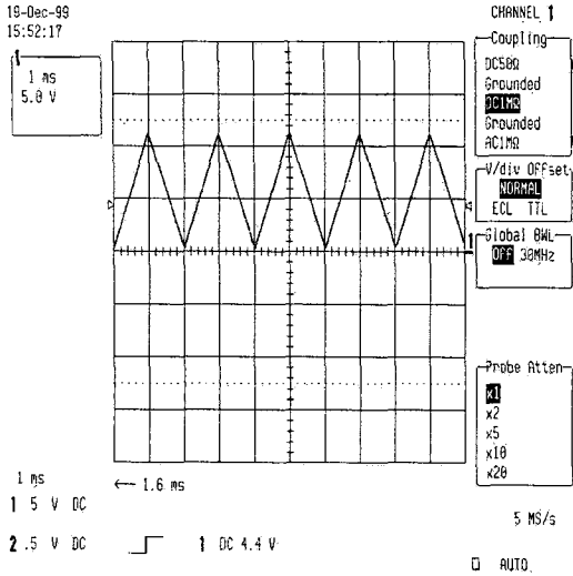
그림 10. 주파수 변조를 하기 위한 삼각파 신호(500 Hz)
