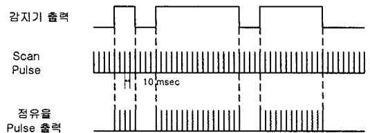
그림 A-3. 감지기의 데이터 스캔 주기
