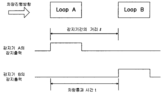
그림 A-1. 속도감지를 하기 위한 Loop A와 Loop B의 펄스 형태
