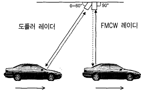
그림 1. 레이더방식 차량감지기 시스템의 설치모양 Fig. 1. Installation and basic operation mode of radar vehicle detector system.
