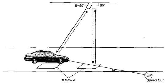
그림 13. 성능측정을 위한 측정시스템 설치
