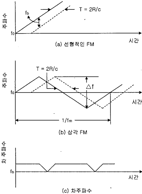
그림 3. 고정된 목표물에 대한 FMCW식의 거리측정 방법을 묘사한 시간대 주파수의 관계 Fig. 3. Relationship for the time versus frequency depicting the method of measuring distance for a fixed target.
