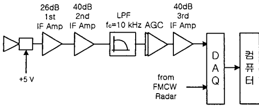
그림 8. 도플러 레이더의 기능적 블록도 Fig. 8. Functional block diagram of Doppler radar.
