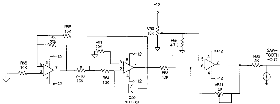
그림 7. 삼각파 발생기 회로도 Fig. 7. Circuit generating triangular wave.
