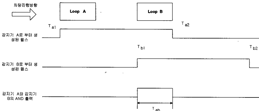
그림 A-2. 차량길이를 감지하기 위한 펄스의 형태
