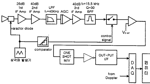
그림 5. FMCW 고도계의 기능적인 블록도 Fig. 5. Functional block diagram of FMCW altimeter.
